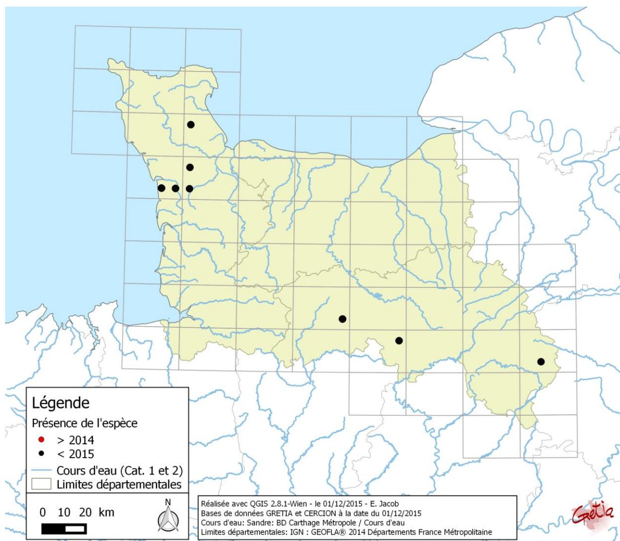
Cartographie des stations connues en Basse-Normandie pour Sympetrum danae
