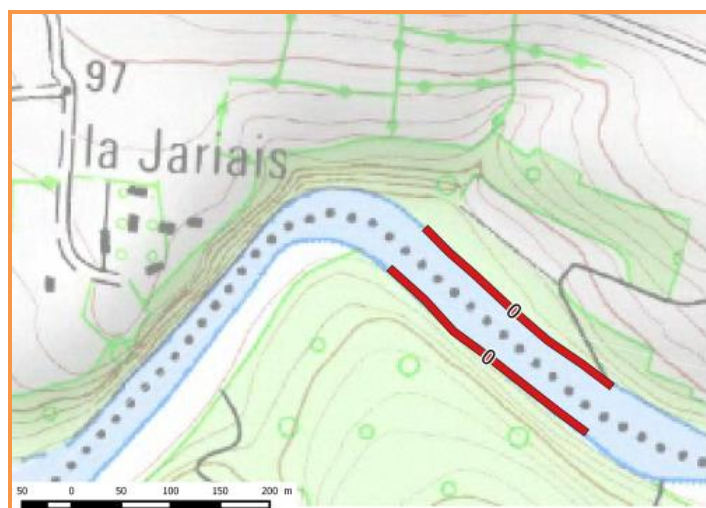
Densités d'exuvies (nb exuvies/100 m. l.) des transects prospectés en 2014 et en 2015 pour Gomphus simillimus en amont des barrages de la Sélune, vers « la Jariais » (aucune variation entre les deux années). D'après LAGARDE (2015).
