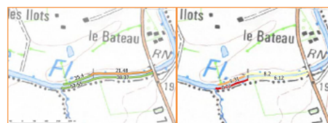
Localisations des transects de prospections pour Gomphus similimus vers « Le Bateau ». Les nombres inscrits sur les transects indiquent la densité d'exuvies de Gomphus similimus récoltées (en nombre d'exuvies par 100 mètres de berges) en 2014 (à gauche) et en 2015 (à droite).
