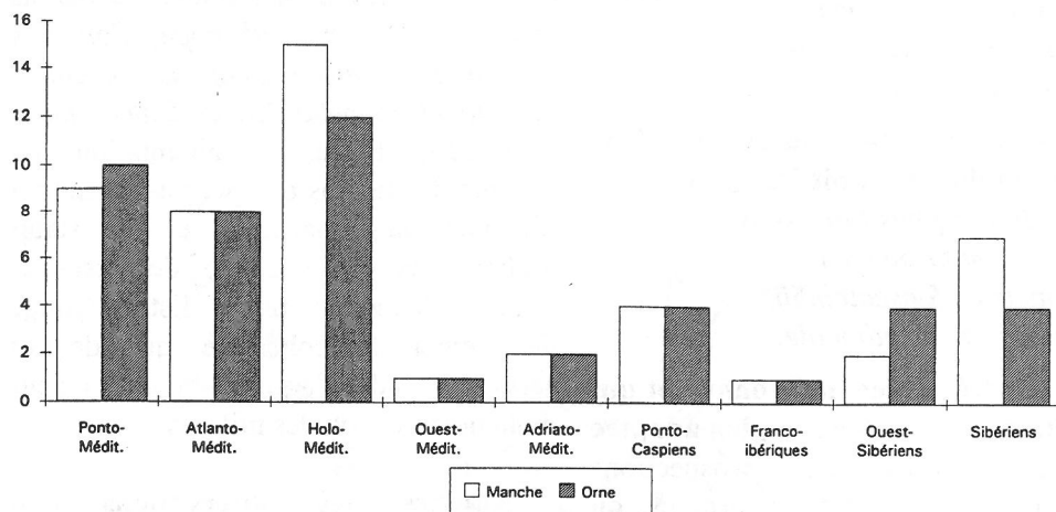
Figure 2.- Compositions comparées des Odonatofaunes des départements de l' Orne (d'après LECOCQ, 1995) et de la Manche. Catégories biogéographiques issues de Devai (1976) in DOMMANGET (1987).
